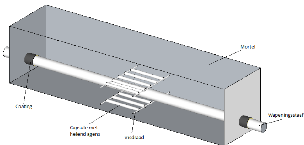
Figuur 3-4: Schetsmatige voorstelling prismatische mortelproefstukken.
