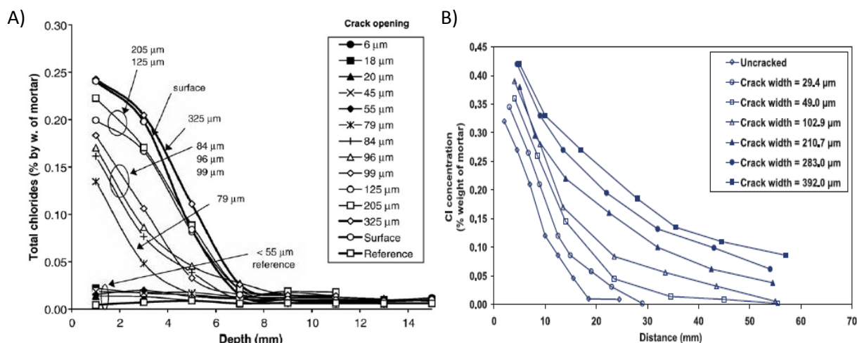
Figuur 2-5: \text{Cl}^- penetratieprofiel loodrecht op de scheur volgens A) Ismaïl et al. en B) Sahmaran & Yaman.
