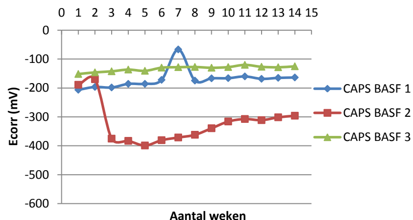
Figuur 4-42: Verloop van E_{\text{corr}} (mV) i.f.v. de tijd (weken) voor met PU MEYCO MP ingekapselde proefstukken, gemeten met de potentiostaat.
