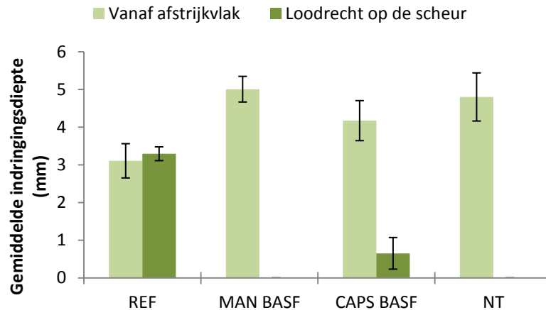
Figuur 4-29: Gemiddelde CO 2 indringingsdiepte gemeten vanaf het afstrijkvlak en loodrecht op de scheur.
