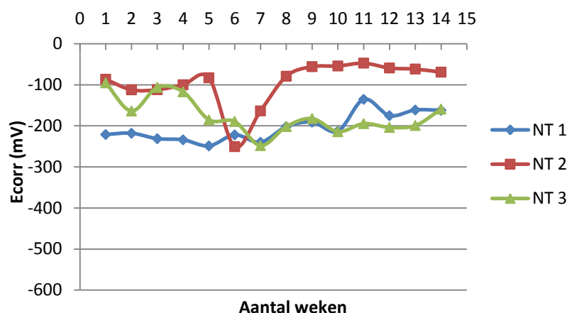
Figuur 4-34: Verloop van E_{\text{corr}} (mV) i.f.v. de tijd (weken) voor de ongescheurde proefstukken, gemeten met de GalvaPulse.
