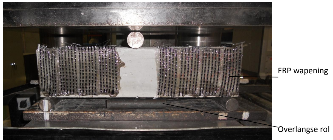
Figuur 3-6: Driepuntsbuigproef.
