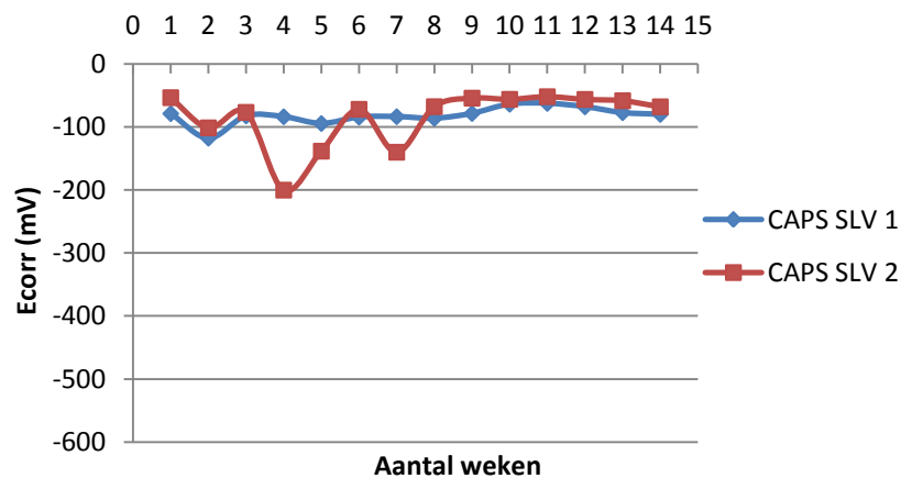
Figuur 4-52: Verloop van E_{\text{corr}} (mV) i.f.v. de tijd (weken) voor met PU flex SLV ingekapselde proefstukken, gemeten met de GalvaPulse.
