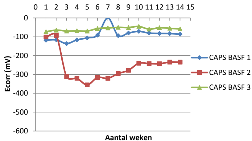
Figuur 4-44: Verloop van E_{\text{corr}} (mV) i.f.v. de tijd (weken) voor met PU MEYCO MP ingekapselde proefstukken, gemeten met de GalvaPulse.
