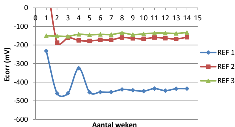
Figuur 4-35: Verloop van E_{\text{corr}} (mV) i.f.v. de tijd (weken) voor de referentie proefstukken, gemeten met de potentiostaat.
