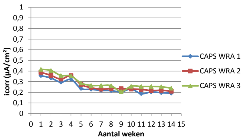
Figuur 4-57: Verloop van i_{\text{corr}} (µA/cm²) i.f.v. de tijd (weken) voor met WRA ingekapselde proefstukken.
