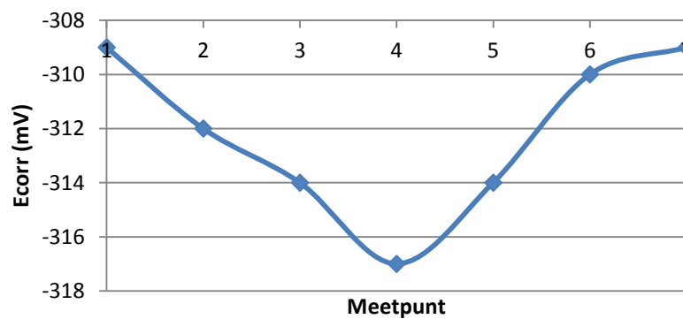
Figuur 4-45: Variatie van E_{\text{corr}} (mV) langsheen balk CAPS BASF 2, gemeten in de 3 e week met de GalvaPulse.
