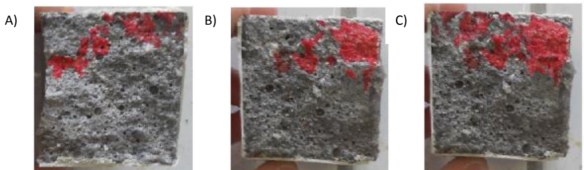
Figuur 4-11: Illustratieve reconstructie van het PU in de scheur voor een proefstuk uit reeks MAN BASF 2.
