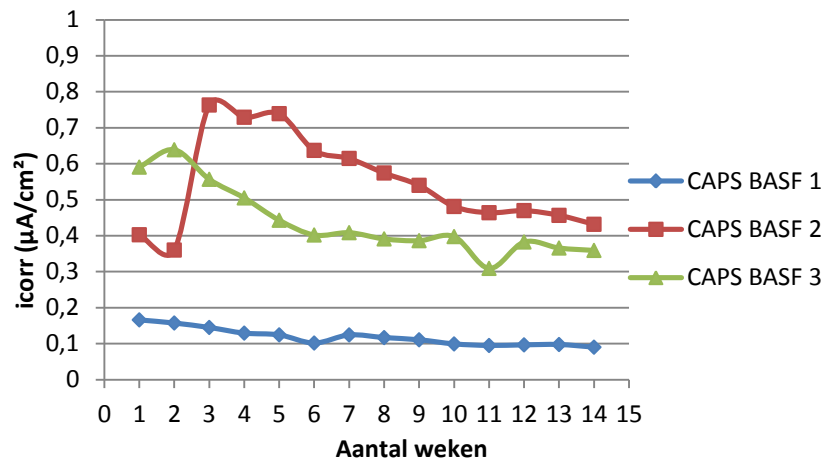
Figuur 4-43: Verloop van i_{\text{corr}} ( \mu\text{A}/\text{cm}^2 ) i.f.v. de tijd (weken) voor met PU MEYCO MP ingekapselde proefstukken.
