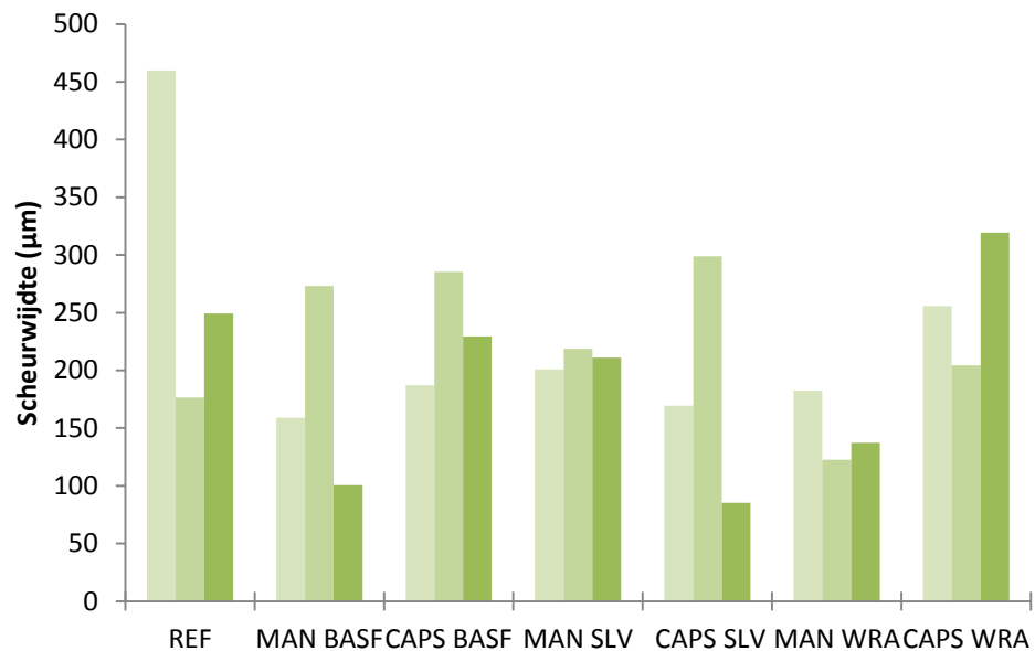
Figuur 4-13: Scheurwijdtes per proefstuk binnen elke reeks.
