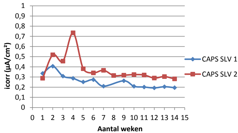
Figuur 4-51: Verloop van i_{\text{corr}} (µA/cm²) i.f.v. de tijd (weken) voor met PU flex SLV ingekapselde proefstukken.
