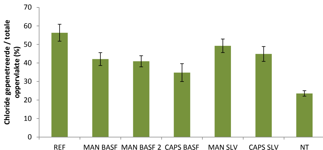
Figuur 4-5: Gemiddelde procentuele verhouding van de oppervlakte waarin chloriden binnengedrongen zijn op de totale oppervlakte voor iedere proefreeks.
