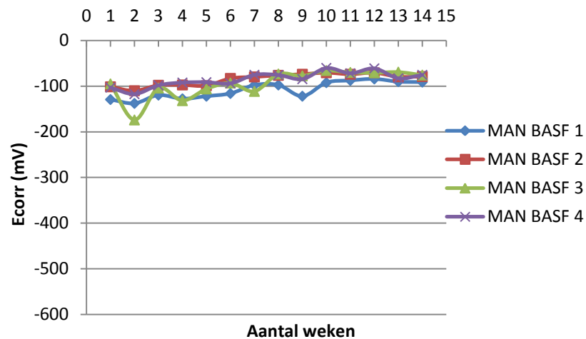
Figuur 4-41: Verloop van E_{\text{corr}} (mV) i.f.v. de tijd (weken) voor manueel met PU MEYCO MP geheelde proefstukken, gemeten met de GalvaPulse.
