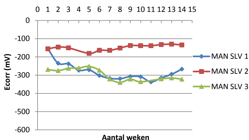
Figuur 4-46: Verloop van E_{corr} (mV) i.f.v. de tijd (weken) voor de manueel met PU flex SLV geheelde proefstukken, gemeten met de potentiostaat.
