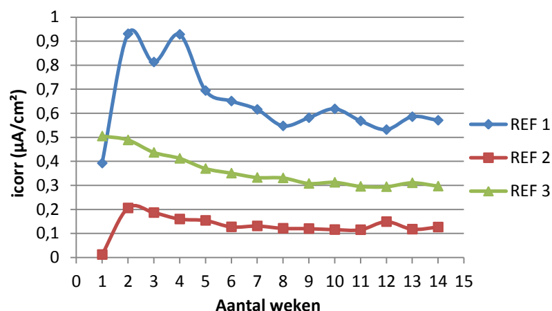
Figuur 4-36: Verloop van i_{corr} (µA/cm²) i.f.v. de tijd (weken) voor de referentieproefstukken.
