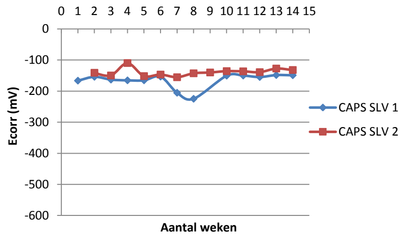
Figuur 4-50: Verloop van E_{\text{corr}} (mV) i.f.v. de tijd (weken) voor met PU flex SLV ingekapselde proefstukken, gemeten met de potentiostaat.
