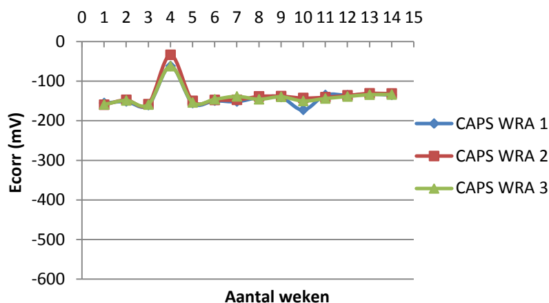
Figuur 4-56: Verloop van E_{\text{corr}} (mV) i.f.v. de tijd (weken) voor met WRA ingekapselde proefstukken, gemeten met de potentiostaat.
