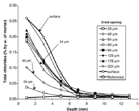
Figuur 2-7: Chloride penetratieprofiel, loodrecht op de scheur die werd vervaardigd na 2 jaar. (Ismail et al. (2008))
