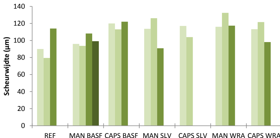
Figuur 4-31: Scheurwijdte van ieder proefstuk per proefreeks.
