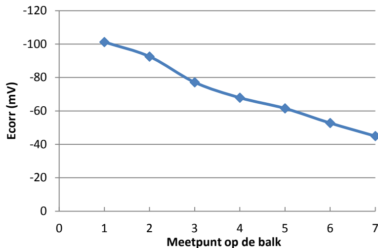
Figuur 3-19: Illustratie van de gevolgen van de polarisatie na toepassen van de galvanostatische pulsmeting.
