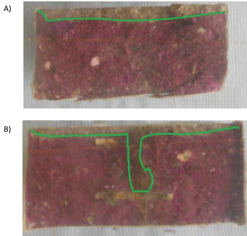
Figuur 4-26: Classificatie van de afgetekende carbonatatieprofielen: A) Equidistante indringing \text{CO}_2 , B) Additionele \text{CO}_2 indringing aan de scheur.
