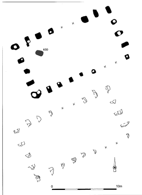
Fig. 156: Grondplan van gebouw 14 (schaal 1/200 e ).
