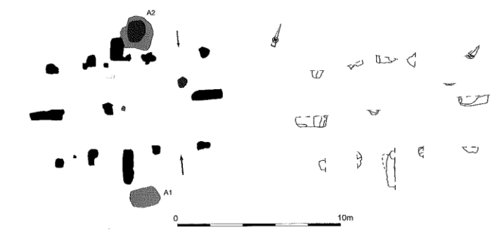
Fig. 117: Gebouw 1 (schaal 1/200 e ).
