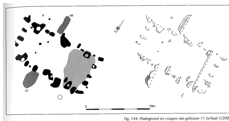
Fig. 144: Plattegrond en coupes van gebouw 11 (schaal 1/200').
