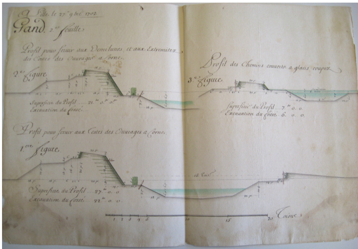
Figuur 6 Plannen voor de uitbreiding van de Gentse versterkingen (Vauban, Rijsel, 27 november 1702)
