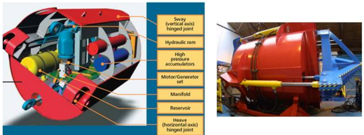
Figuur II-4: Conversiemodule van de Pelamis [14]
