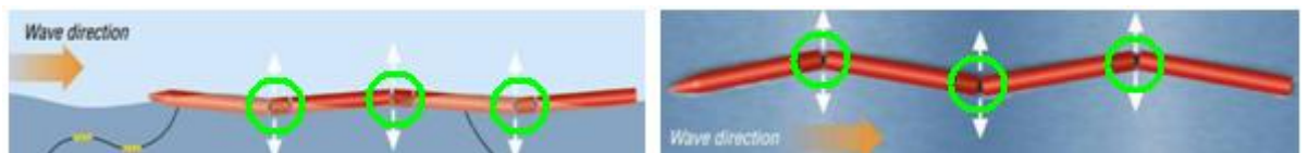
Figuur II-5: De drie conversiemodules van de Pelamis in zij- en bovenaanzicht [18]
