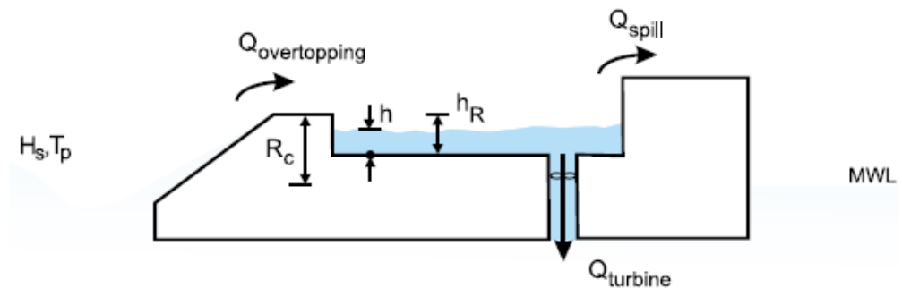
Figuur II-14: Werkingsprincipe van de Wave Dragon [27]
